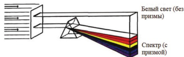
Рис. 63: Расщепление белого солнечного луча света в различные цвета, как было продемонстрировано в эксперименте Исааком Ньютоном в 1676 г.
