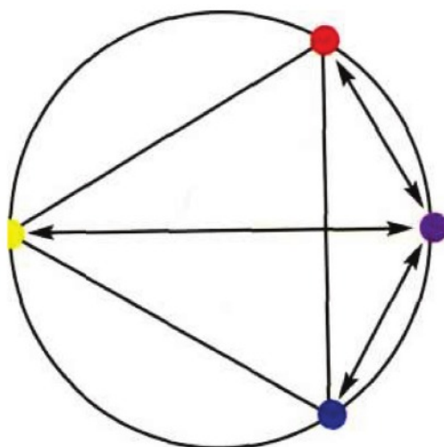
Рис. 82: Фиолетовый связан с тремя основными цветами. Это смешение красного и синего и дополнительный цвет желтого.
