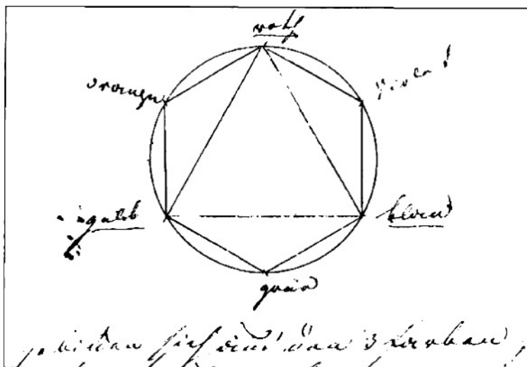
Рис. 64: Цвета радуги, расположенные по кругу И.В.Гете. Из О. Kratz (ed.), Goethe und die Naturwissenschaften, сmp. 174.
