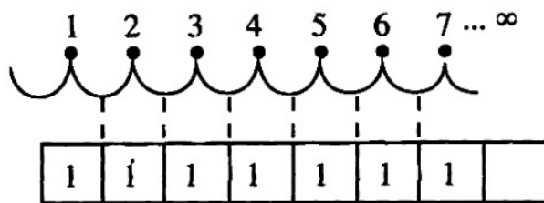
Рис. 91: Число «1» как единичное число и основа всех натуральных чисел.
