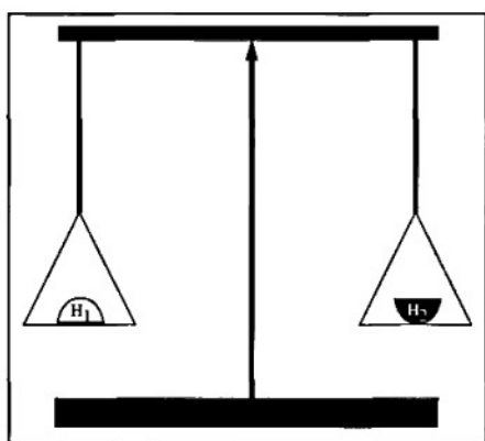
Рис. 26. Две гипотезы на весах. Любое усиление критерия обосновывает или гипотезу (H1) или контргипотезу (H2) и, таким образом, показывает, какой стороне дано больше подтверждений.
