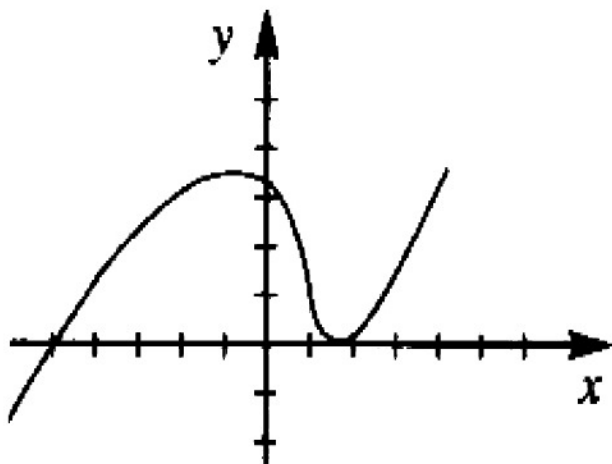
Рис. 103: Декартов крест
